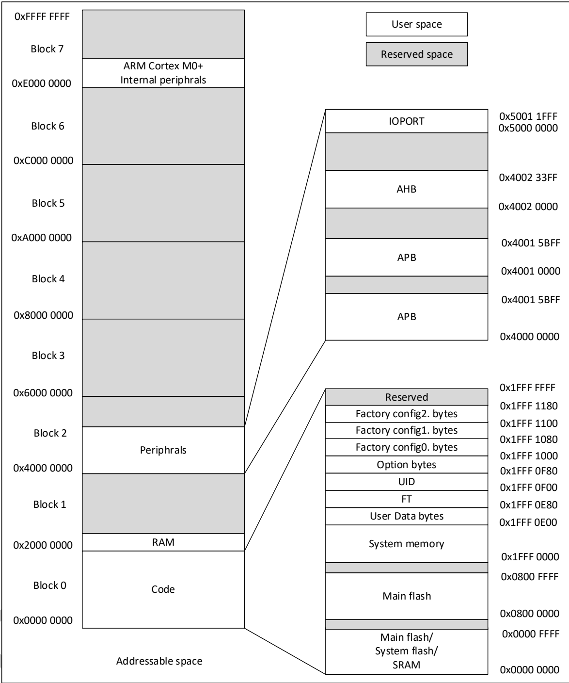
图 4-1 存储器映射
