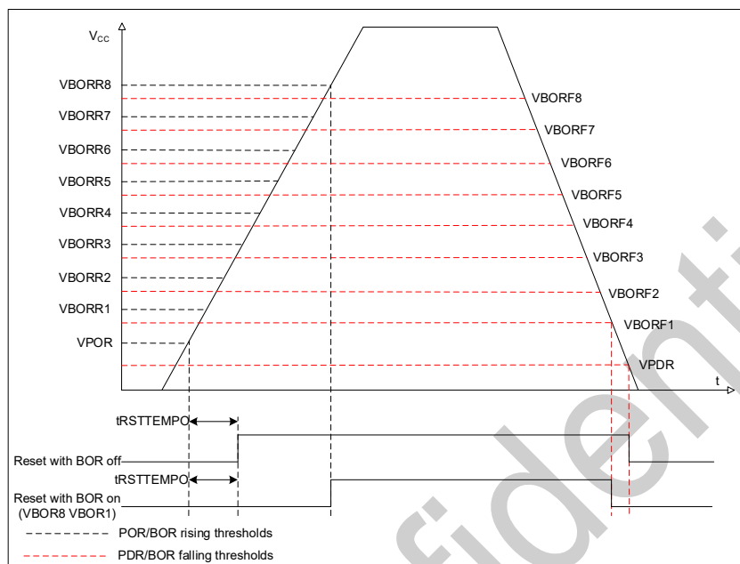
图 2-4 POR/PDR/BOR 阈值
