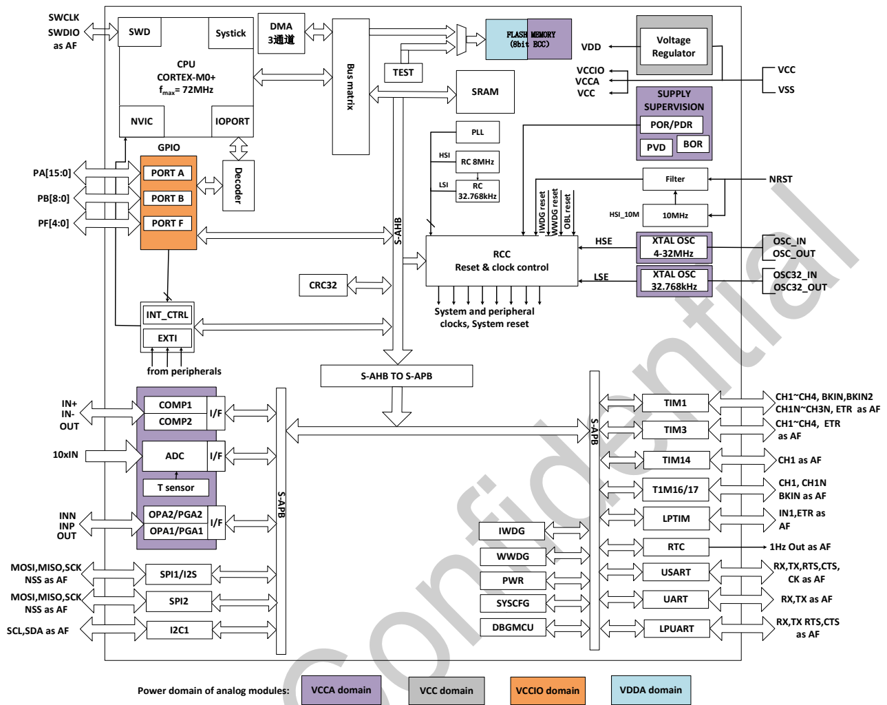
图 1-1 功能模块
